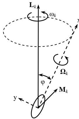
Рис. 3. Прецессия волчка.
