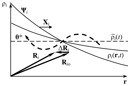
Рис. 2. К образованию вектора поляризации.
