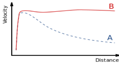
Рис. 4. Кривые вращения галактик
