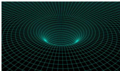
Рис.5. Иллюстрация «гравитационной воронки» в ОТО
