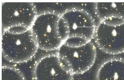
Рисунок 3. Участок карты Вселенной с изображением кольцевых структур (Source: Berkeley National Laboratory)
