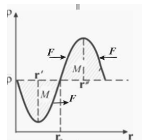
Рис. 4. Силы «тяготения» и «отталкивания»
